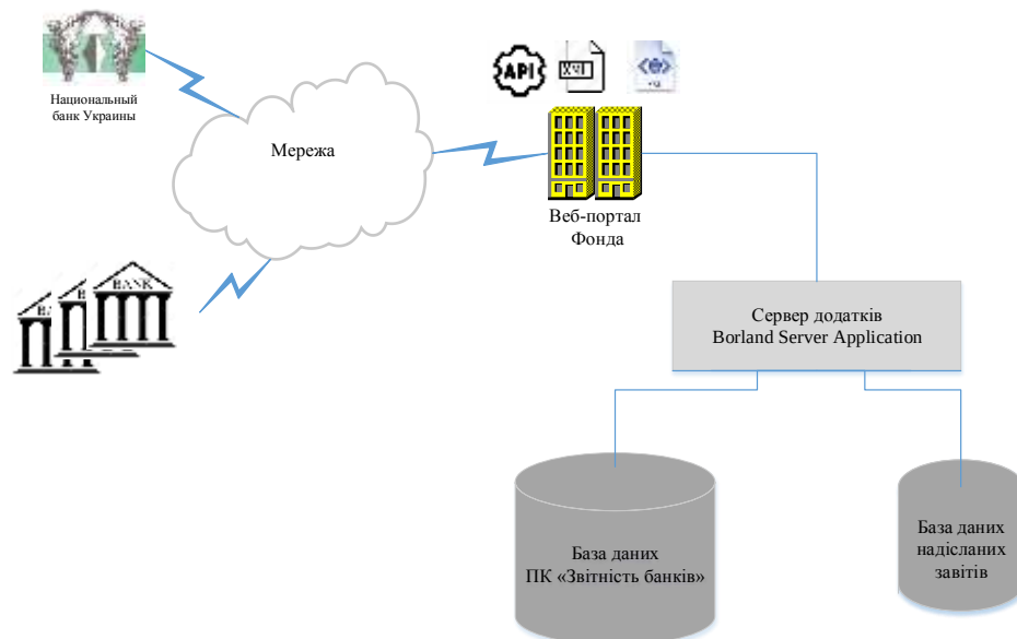
Рис. 9.5. Схема застосування XML-звітності
