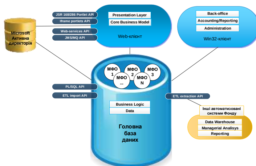
Рис. 9.3. Складові частини ЄОІС
