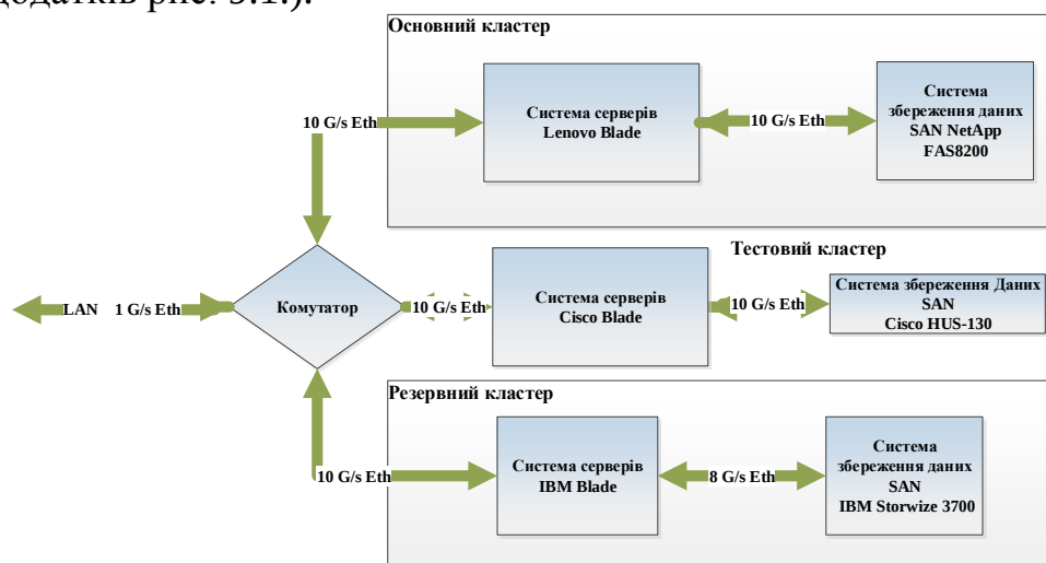
Рис. 9.1. Програмно-апаратний комплекс Фонду
