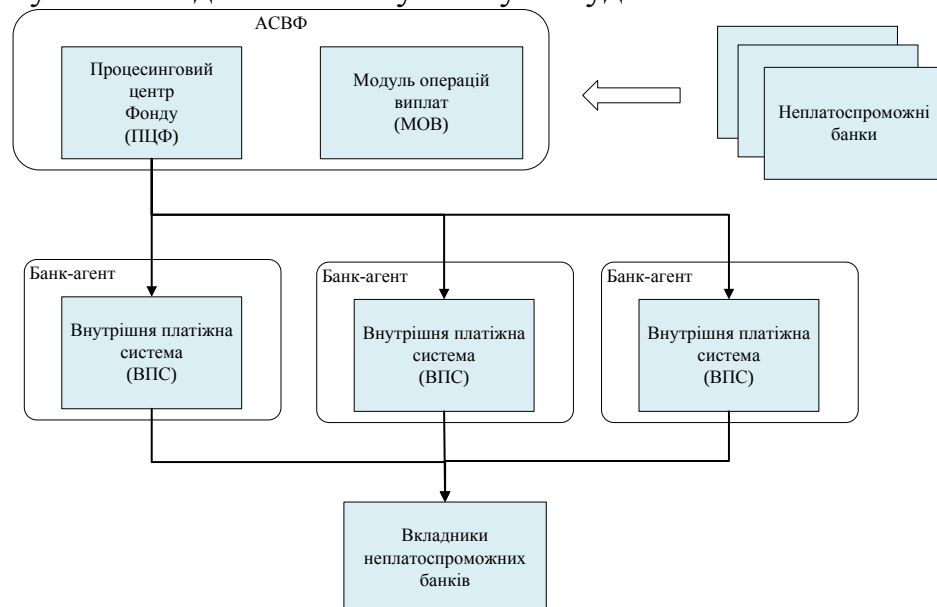
Рис. 9.4. Автоматизована система виплат Фонду
