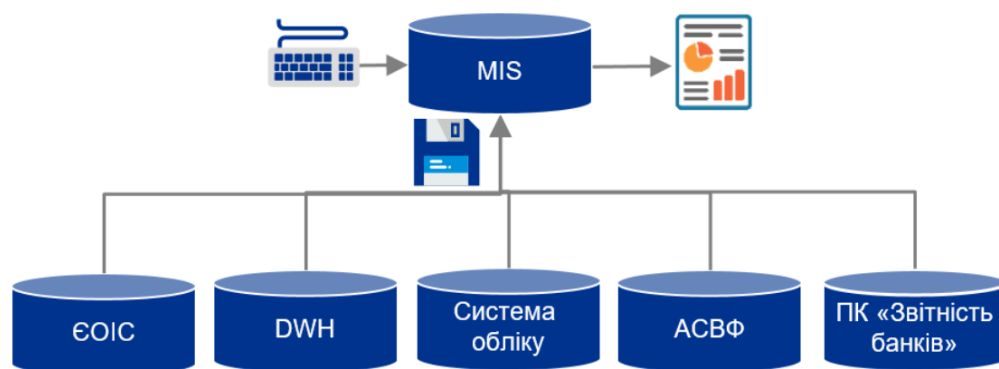
Рис. 9.4.1. Системи аналізу даних та аналітичної звітності (MIS)
